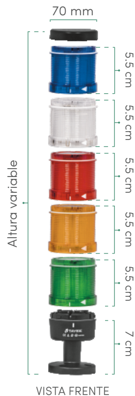
VISTA FREENTE
