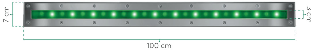
VISTA FRENTE LEDs Verdes encendidos
