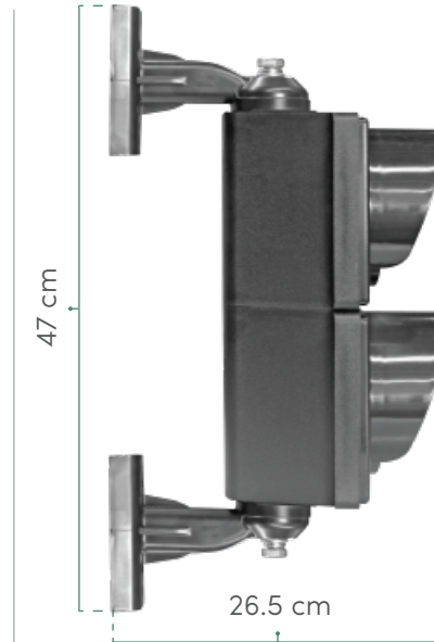
VISTA IZQUIERDA Con brazos de montaje.
